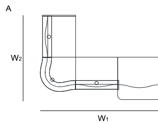
A: LUV06L + LUV01 + LUV07L + LUV03 02 + LUV04 + LUV03 02 + LUV05P B: LUV05L + LUV03 02 + LUV04 + LUV03 02 + LUV07P + LUV01 + LUV06P
