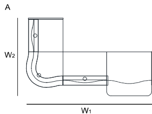
A: LUV06L + LUV01 + LUV07L + LUV03 + LUV04 + LUV02 + LUV05P B: LUV05L + LUV02 + LUV04 + LUV03 + LUV07P + LUV01 + LUV06P
