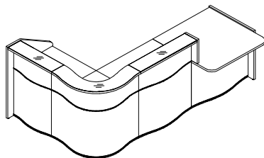
A: LUV06L + LUV01 + LUV07L + LUV03 + LUV04 + LUV02 + LUV05P B: LUV05L + LUV02 + LUV04 + LUV03 + LUV07P + LUV01 + LUV06P
